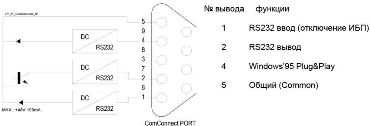
Рис. 7 – Порт ComConnect
