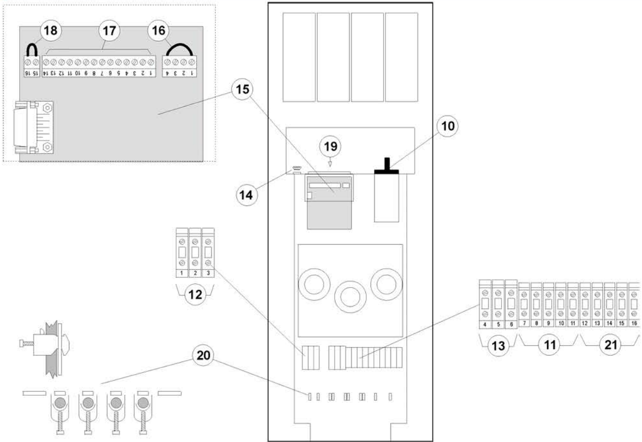
Рис.6 – Задняя панель
